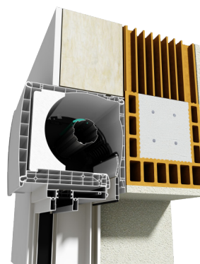
COFFRE ISOFT
